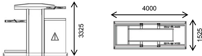
Jet-Fill Big Bag Filler
