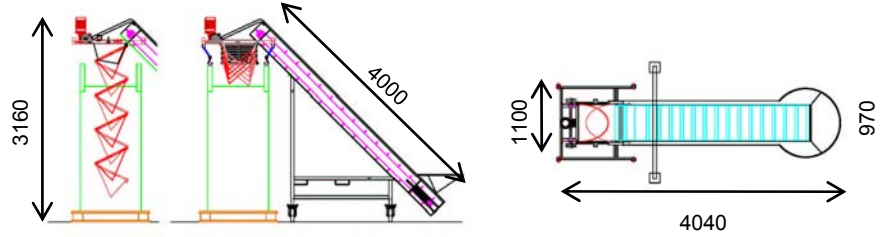
Solo-Fill Big Bag Box Filler
